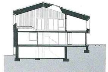
Querschnitt | Section
